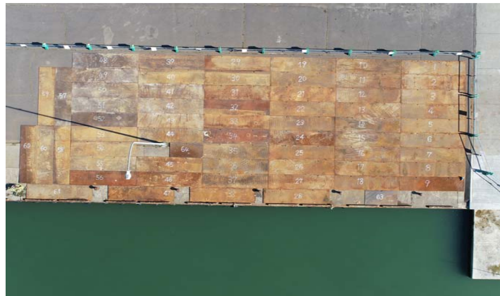
撮影年月日 令和7年8月28日 岸壁保護 敷鉄板設置完了 全64枚
