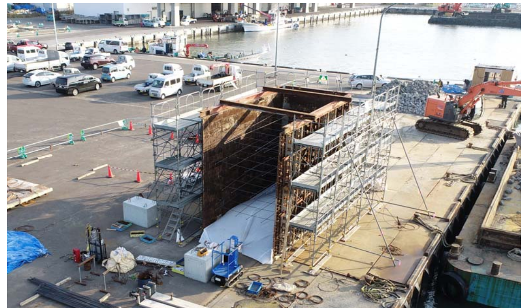
撮影年月日 令和7年10月31日 -3.5m岸壁 本体工[場所打式] 型枠組立状況
